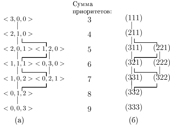
Рис. 4.7. Два представления решетки качества e(S)
