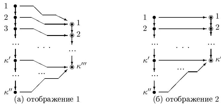
Рис. 3.14. Порядковая шкала \Rightarrow порядковая
