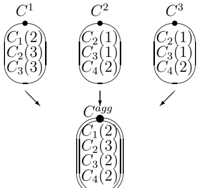
Рис. 18.9. Агрегация для C
