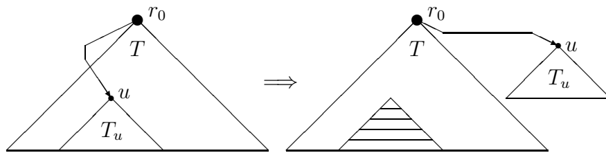
Рис. 6.24. Задача горячей связи (одна связь)
