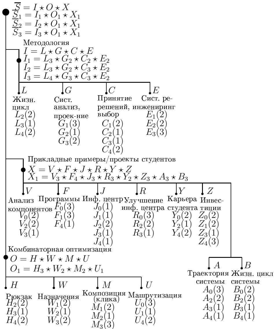
Рис. 18.23. Надструктура для агрегированного курса (структура \bar{\Lambda} )
