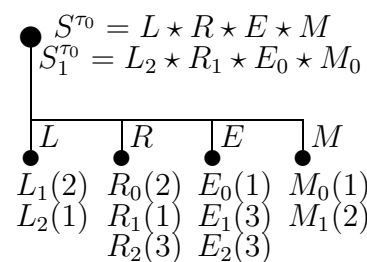
Рис. 8.9. Структура группы ( \tau_0 )
