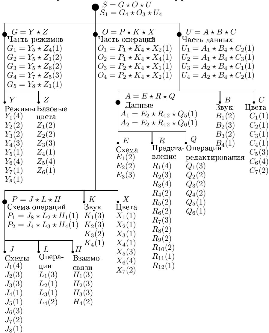
Рис. 10.7. Иерархическая схема фрагмента пользовательского интерфейса (приоритеты для DAs указаны в скобках)
