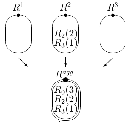
Рис. 18.18. Агрегация для R
