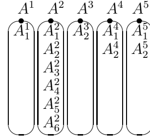
Рис. 17.8. Надструктура
