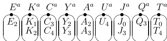
Рис. 9.6. Надрешение
