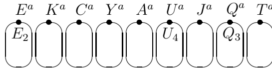
Рис. 9.7. Подрешение
