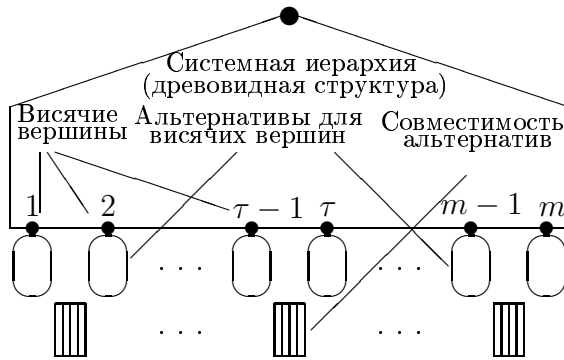
Рис. 1.7. Системная морфология
