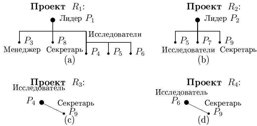
Рис. 11.1. Структура проектов
