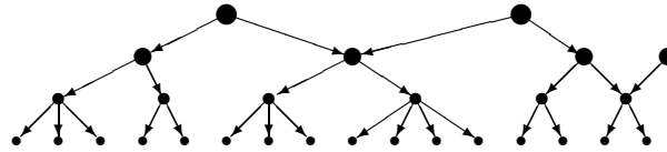
Рис. 1.4. Поли-дерево
