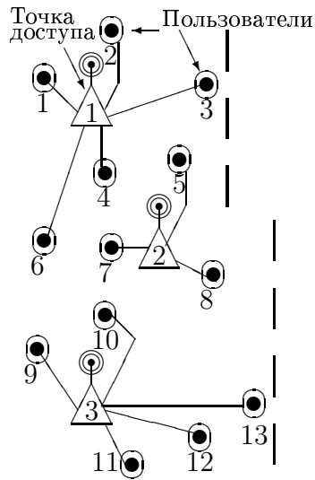
Рис. 13.27. Исходный регион
