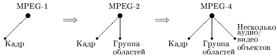
Рис. 13.14. Видео кодирование (2.1.1)
