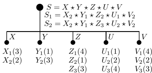
Рис. 6.16. Пример системы
