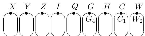
Рис. 16.6. Подрешение
