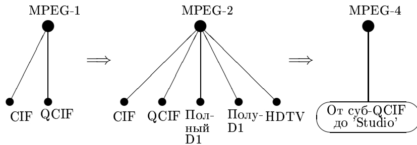
Рис. 13.12. Резолюция (1.3.1)
