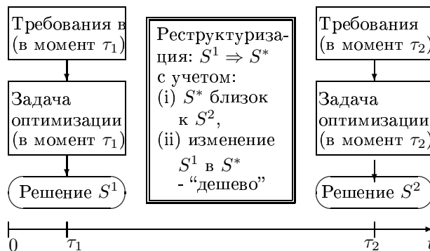
Рис. 6.14. Процесс реструктуризации [350]
