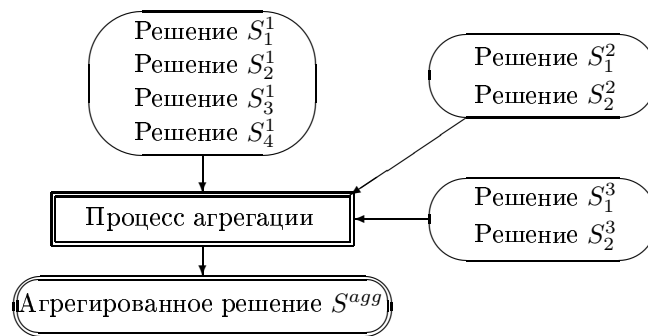
Рис. 18.5. Агрегация решений
