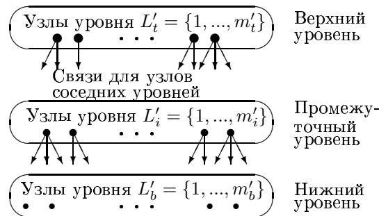
Рис. 5.10. Многоуровневые структуры
