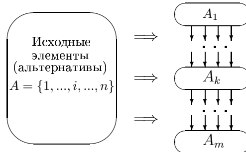
Рис. 7.11. Схема ранжирования
