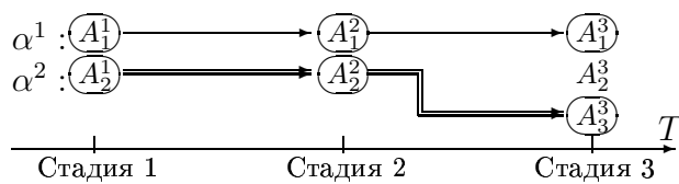
Рис. 13.20. Траектории изменения
