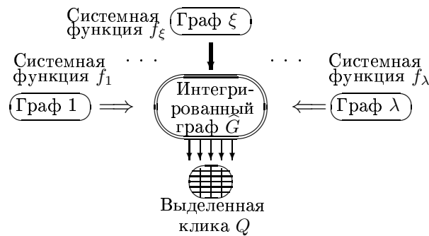
Рис. 5.18. Выявление клики
