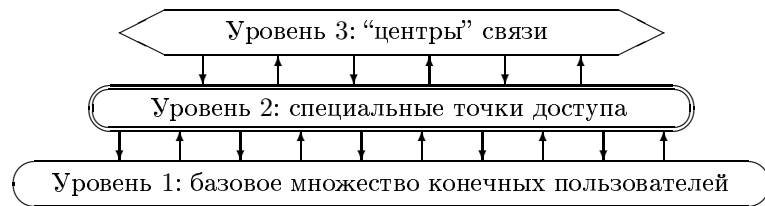
Рис. 2.9. Трех-уровневая модель сети
