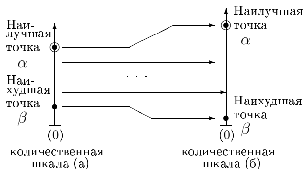
Рис. 3.12. Трансформация количественной шкалы
