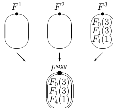
Рис. 18.16. Агрегация для F
