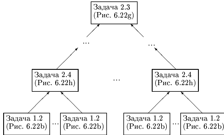
Рис 6.23. Схема 'СНИЗУ-ВВЕРХ' для древовидного графа [334]
