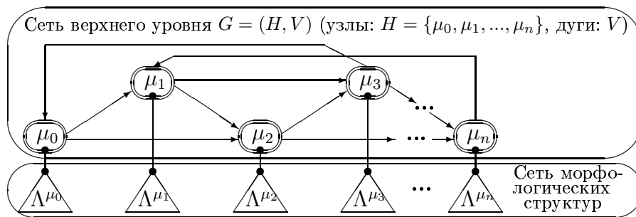
Рис. 1.9. Двух-уровневая модель: сеть с морфологиями
