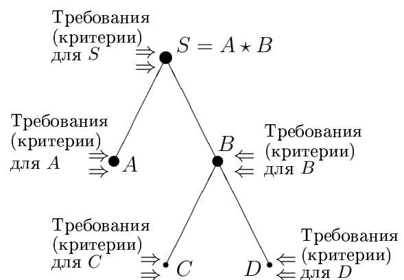
Рис. 4.6. Иерархия требований
