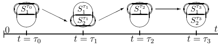
Рис. 8.14. Траектория группы
