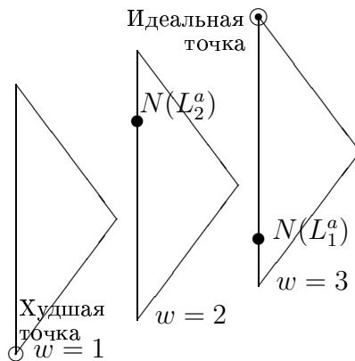
Рис. 9.5. Качество L^a
