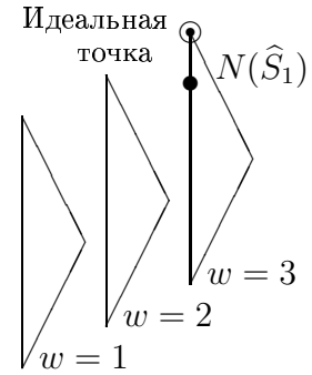
Рис. 12.9. Качество \hat{S}
