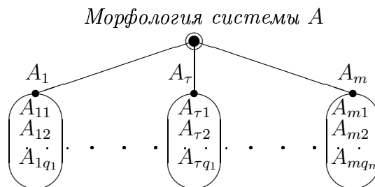
Рис. 7.13. Морфология системы
