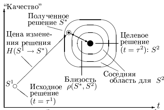
Рис. 6.15. Задача реструктуризации [350]
