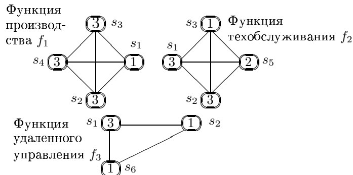
Рис. 5.16. Упрощенный пример
