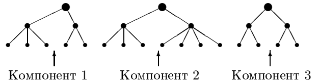
Рис. 1.3. Лес
