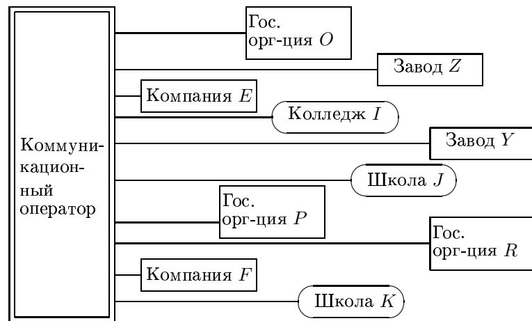
Рис 13.1. Иллюстративная схема
