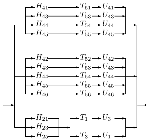
Рис. 10.15. Последовательно-параллельные стратегии
