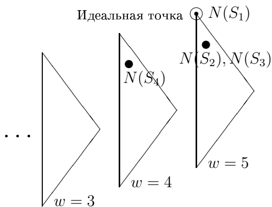
Рис. 17.17. Решетка качества
