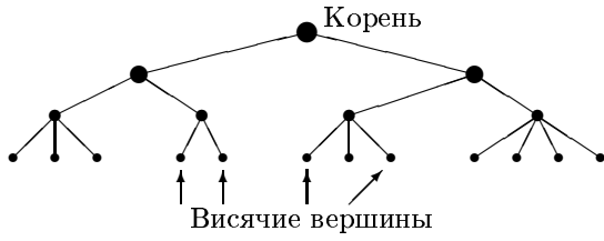
Рис. 1.2. Дерево
