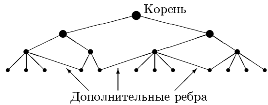
Рис. 1.6. Иерархия
