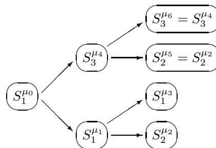
Рис. 8.21. Древоподобная траектория
