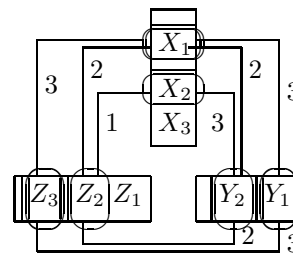
Рис. 4.10. Концентрическое представление
