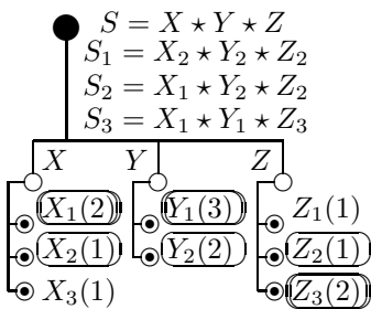
Рис. 4.9. Пример композиции
