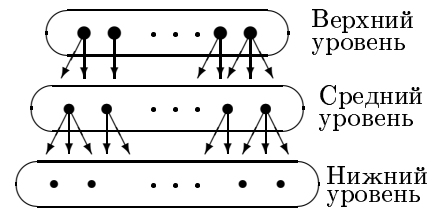
Рис. 1.8. Многоуровневая структура
