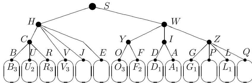
Рис. 7.39. Решение S^{2c}
