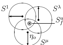
Рис. 7.37. Агрегация [334]
