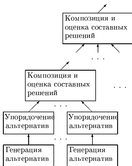
Рис. 4.5. Схема 'снизу-вверх'
