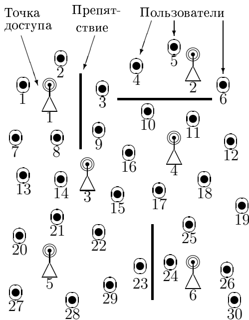
Рис. 13.7. Исходный пример
