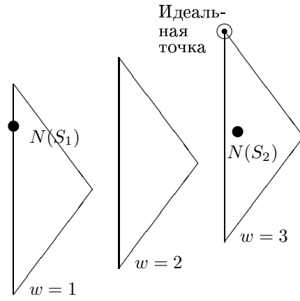
Рис. 6.17. Шкала качества
