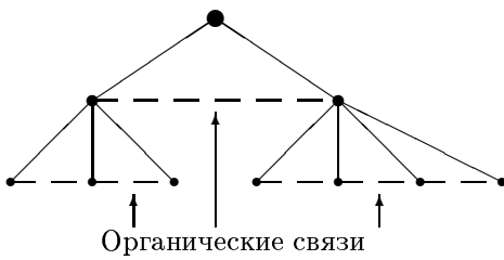
Рис. 1.5. Органическая иерархия
