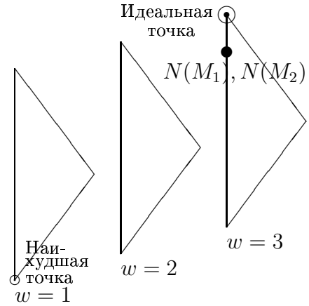
Рис. 16.12. Решетка качества
