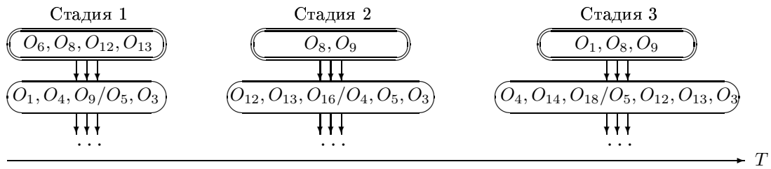
Рис. 13.19. Расширенные множества лучших и 'квази-лучших' операций
